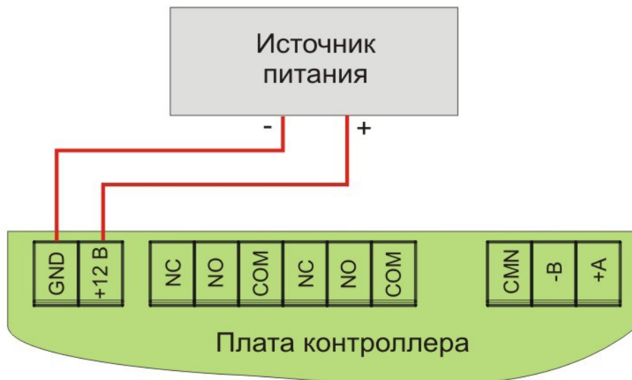
Рисунок 3. Подключение источника питания
