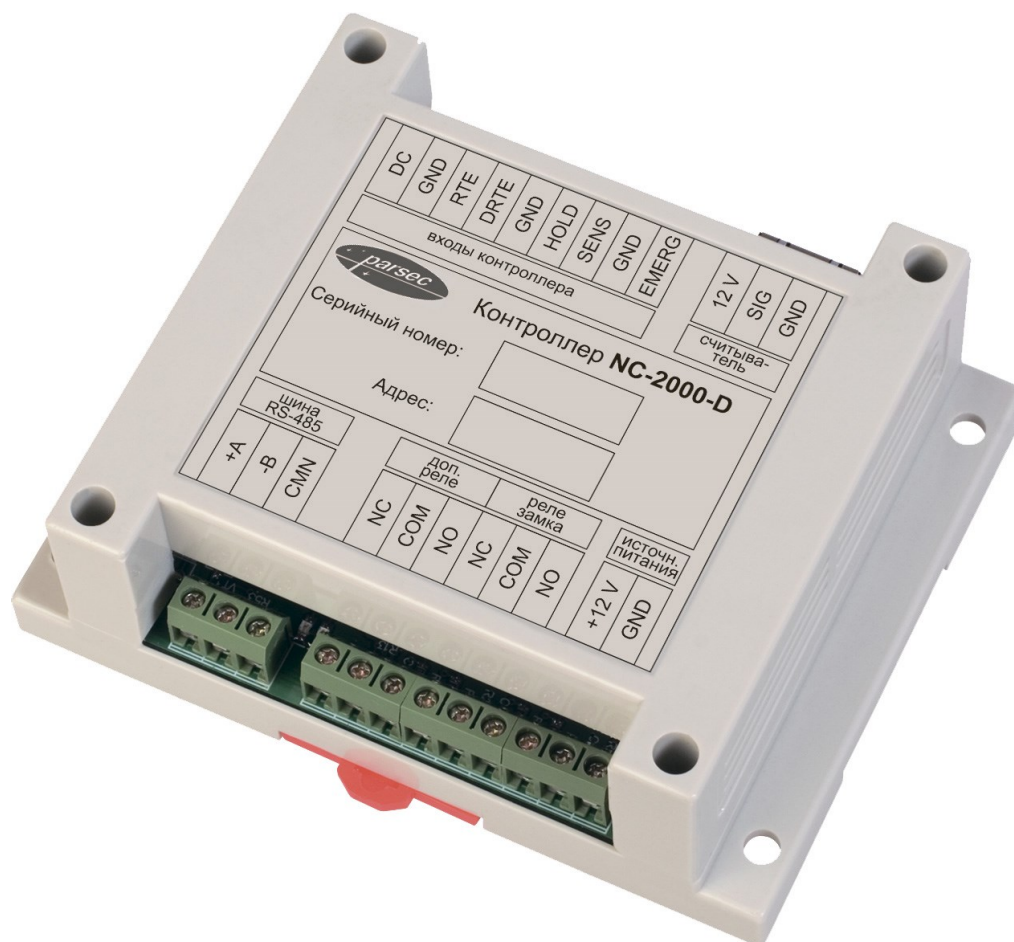
Рисунок 1. Контроллер NC-2000-D в корпусе
