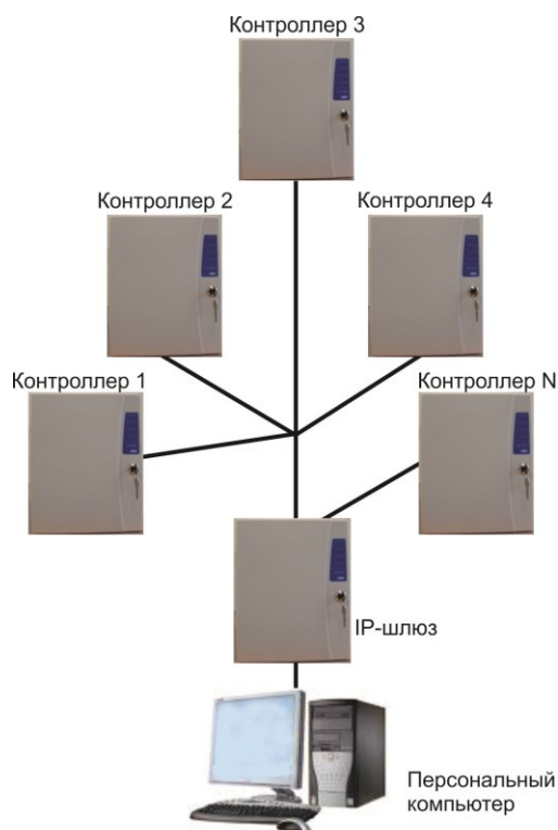
Рисунок 18. Соединение контроллеров по топологии «Звезда»
