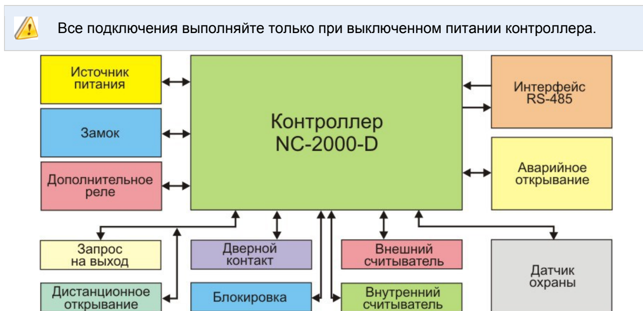
Рисунок 4. Оборудование, подключаемое к контроллеру NC-2000-D
