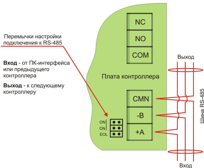
Рисунок 19. Подключение контроллера к шине RS-485
