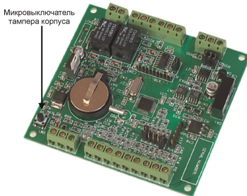
Рисунок 15. Микровыключатель тампера корпуса
