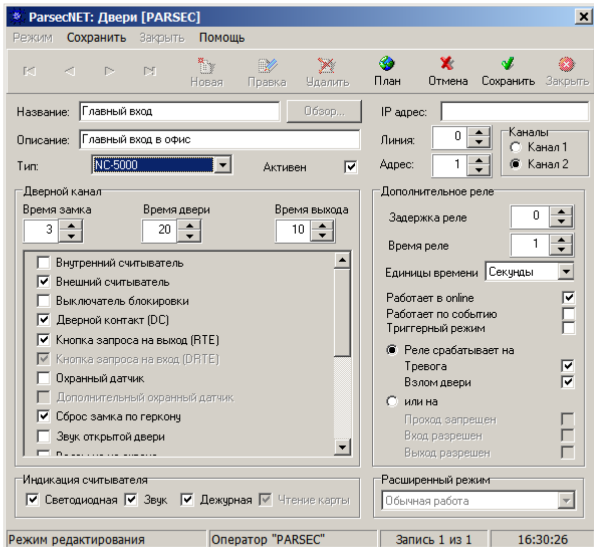
Рисунок 22. Настройка контроллера в ParsecNET 2.5
