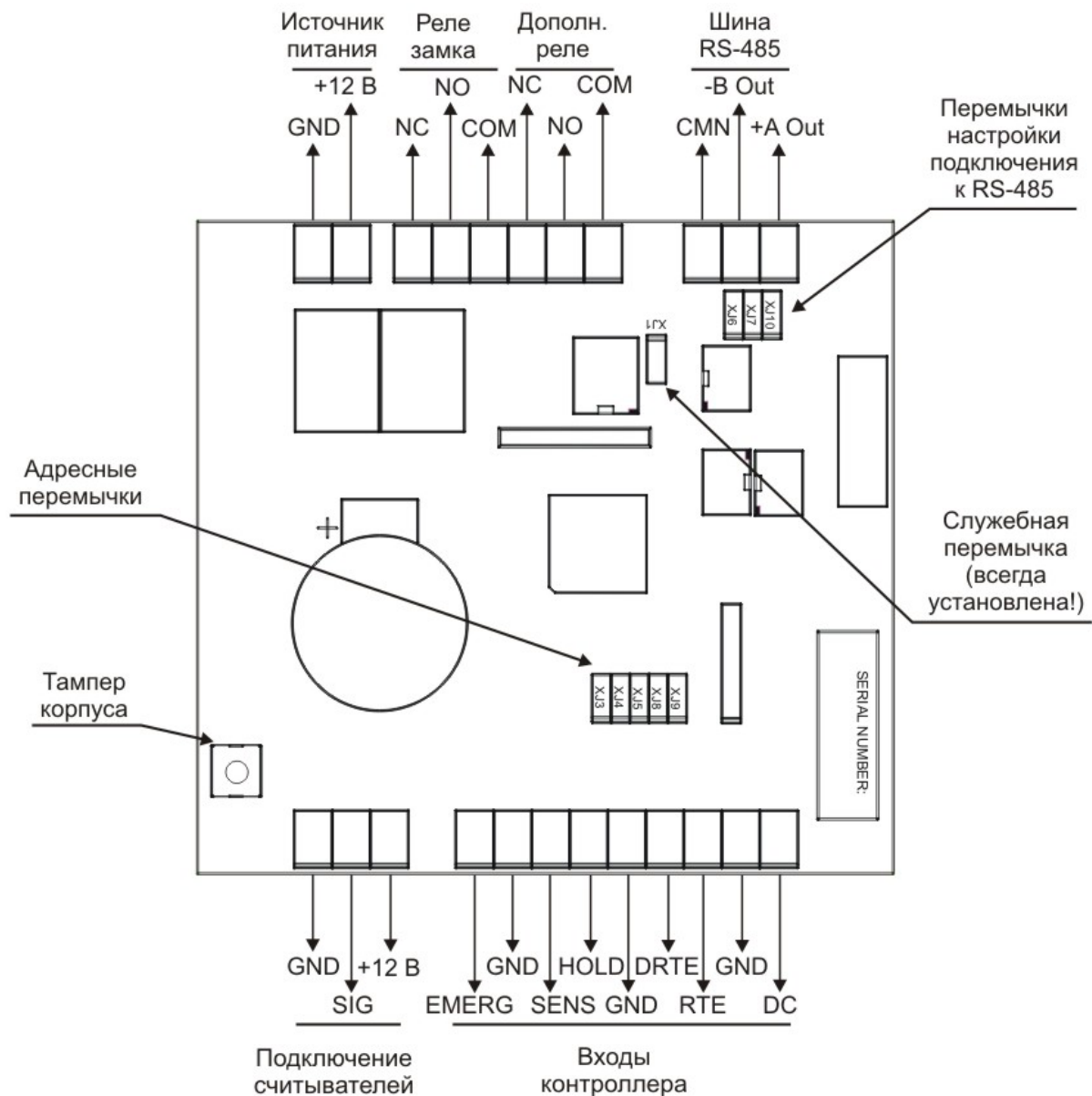
Рисунок 2. Схема платы контроллеров NC-2000D
