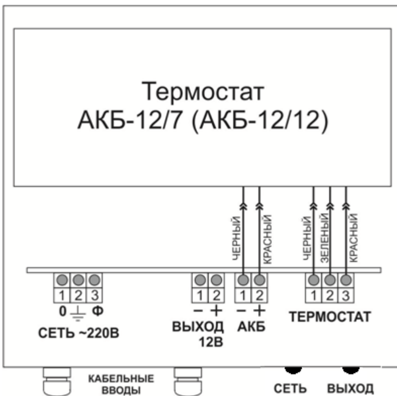
Рисунок 3. Экономичный вариант подключения термостата АКБ к источнику (с отключением термостатирования в режиме «Резерв»)
