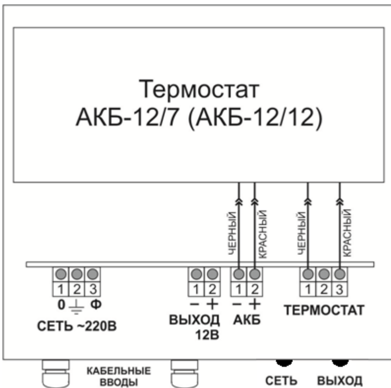
Рисунок 2. Стандартный вариант подключения термостата АКБ к источнику (без отключения термостатирования в режиме «Резерв»)
