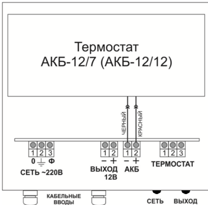
Рисунок 1. Вид источника с открытой крышкой (схема подключения)
