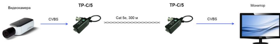
Рис.2 Схема подключения TP-C/5
