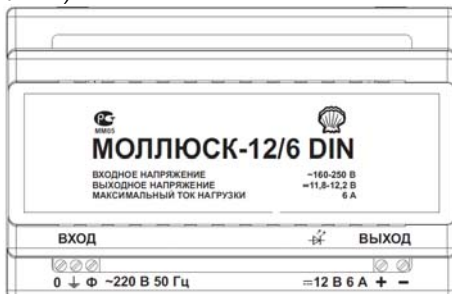
Рис.1. Внешний вид
