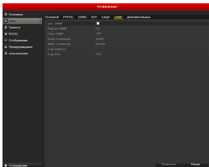
Рис. 9.12 Интерфейс конфигурации SNMP
