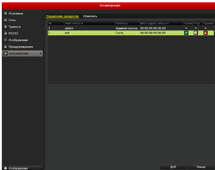
Рис. 13.9 Редактирование пользователя
