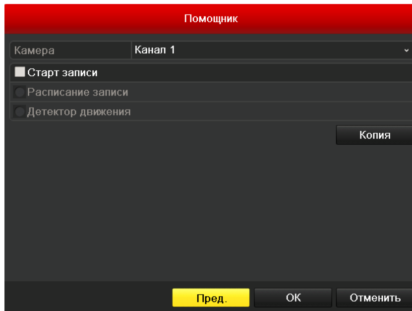
Рис.2.6. Настройка записи
