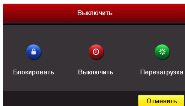
Рис.3.10. Выключение
