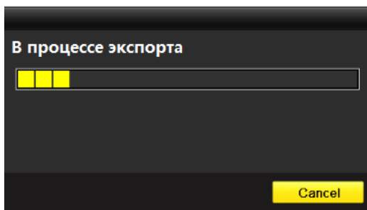
Рис.9.26 Экспорт конфигурации
