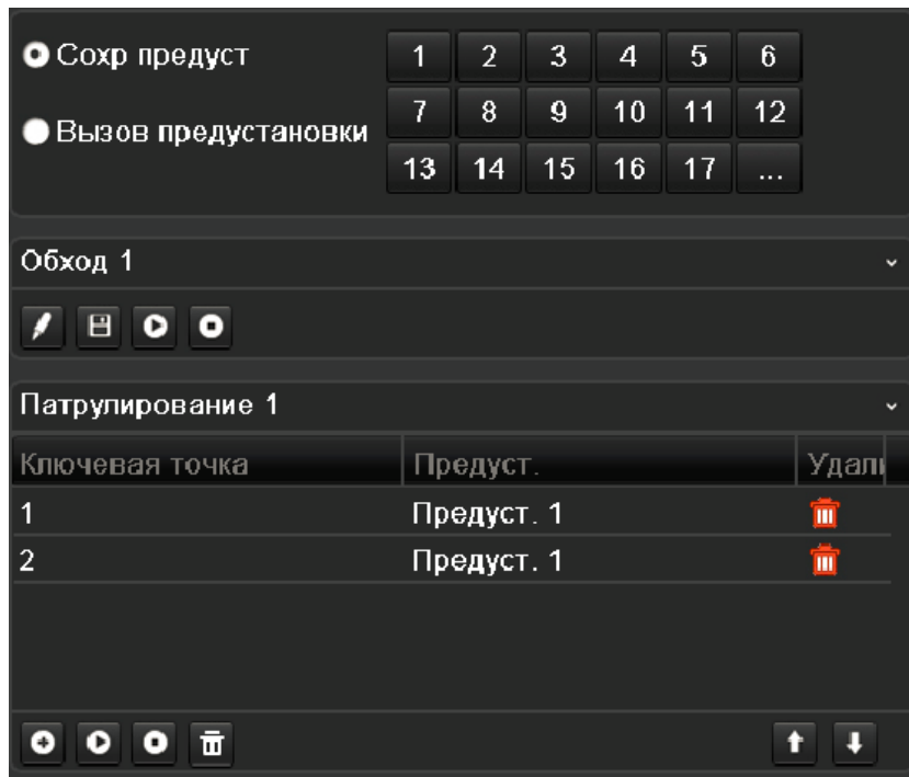
Рис. 4.4 Запуск патруля
