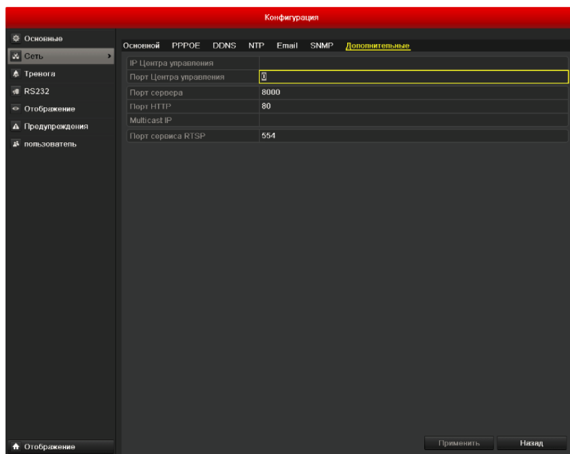
Рис. 9.16 Конфигурация мультикаста
