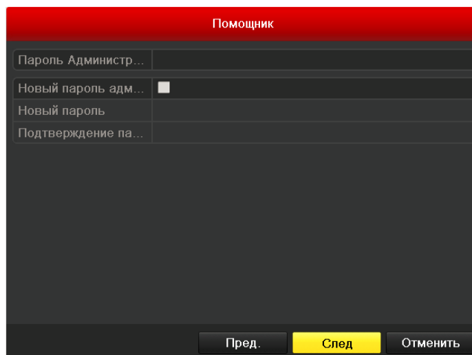
Рис.2.2. Окно входа
