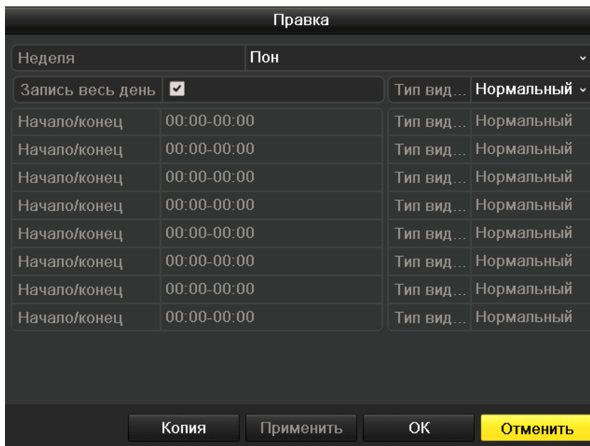
Рис. 5.8 Редактирование расписания
