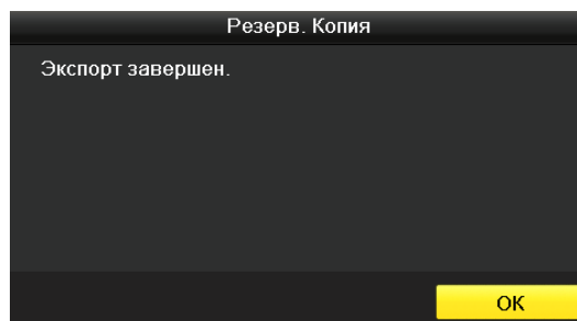
Рис. 7.8 Экспорт завершен
