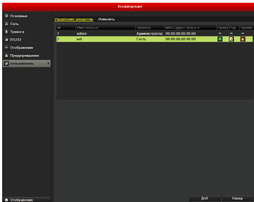
Рис. 13.8 Удаление пользователя
