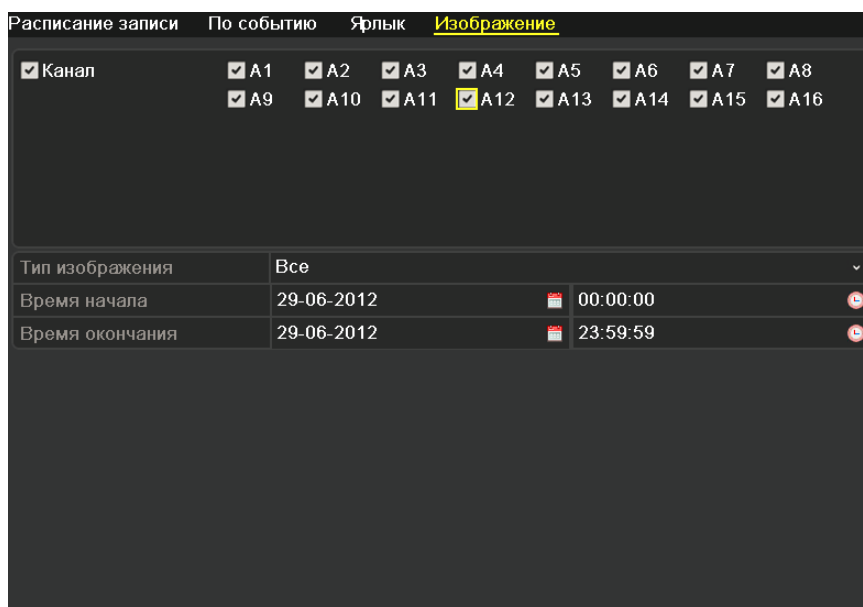
Рис. 6.38 Поиск изображений
