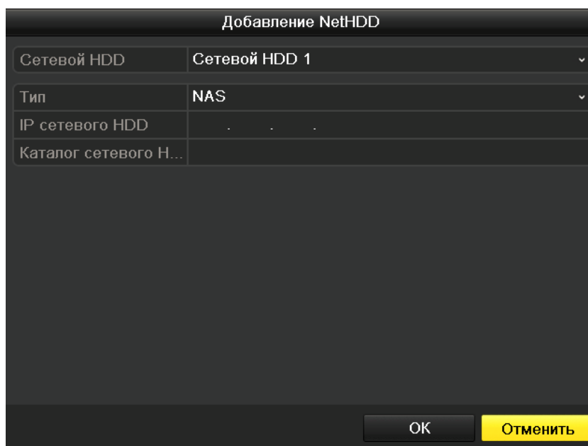
Рис. 10.6 Добавление NetHDD
