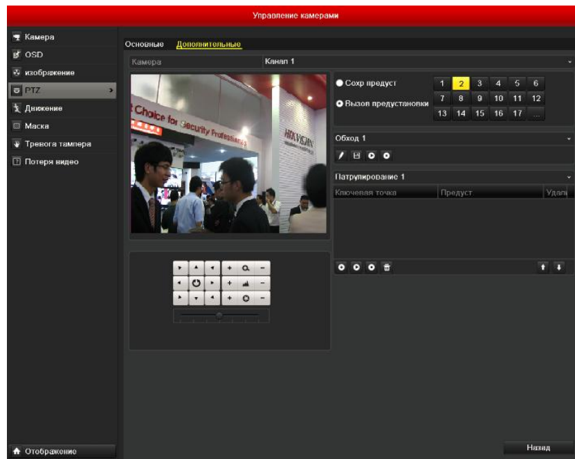
Рис. 4.6 PTZ- шаблоны
