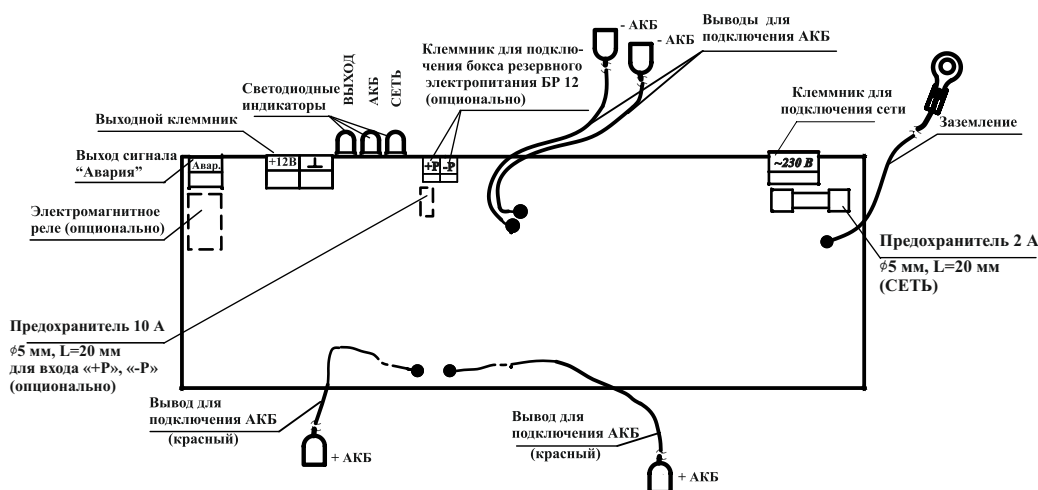
Рисунок 1– Плата источника
