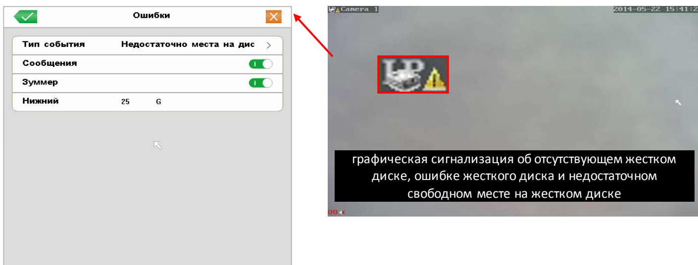
Рисунок № 81 - Подменю «Ошибки» (Слева). Графическая сигнализация (Справа)
