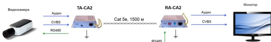
Рис.4 Пассивно-активная передача видео, аудио и данных.
