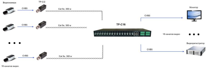
Рис.2 Схема подключения TP-C16
