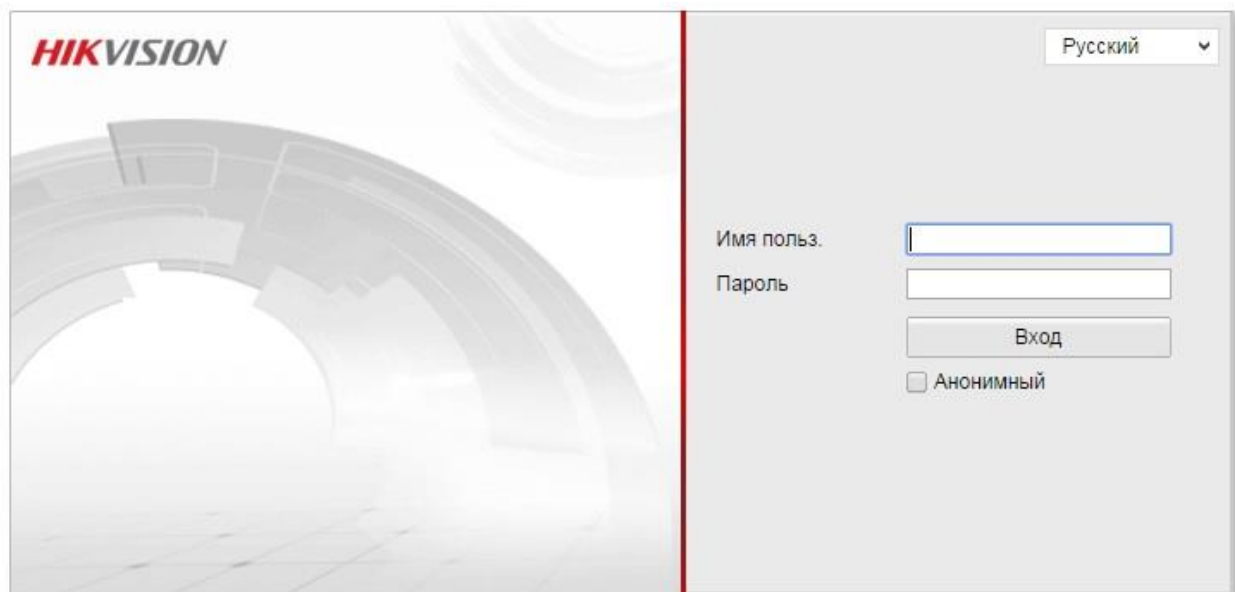
Рисунок 3-1 Окно входа
