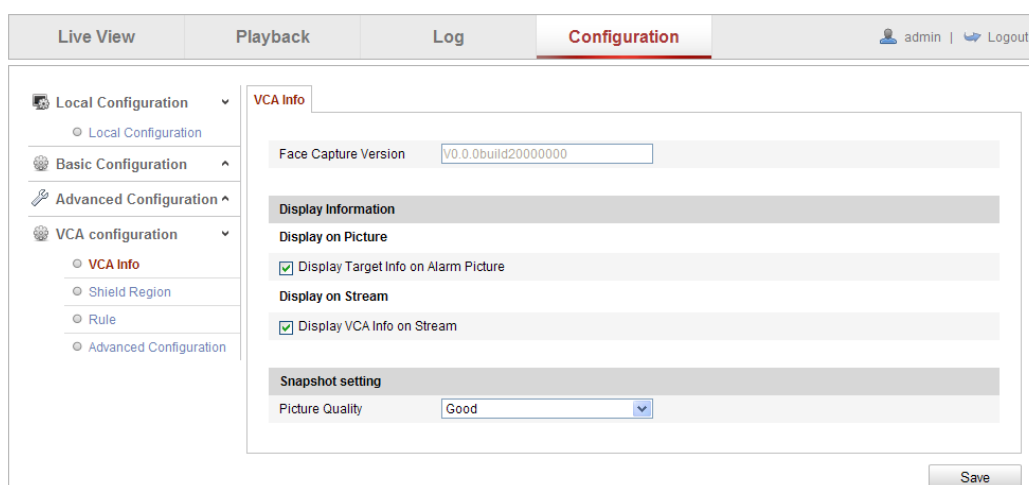
Рисунок 6-51 Захват лица
