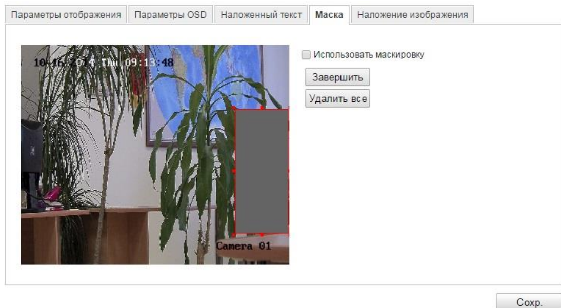
Рисунок 6-31 Настройки маски
