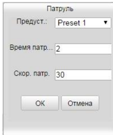
Рисунок 5-6 Настройка патруля
