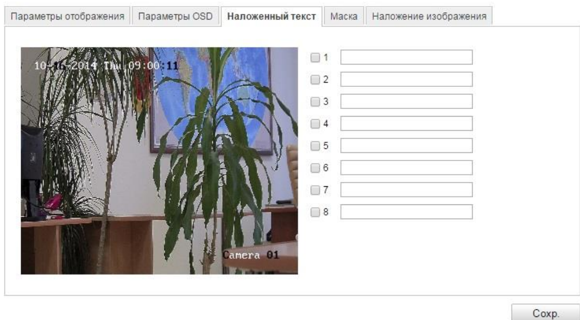
Рисунок 6-30 Наложение текста
