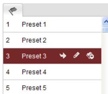
Рисунок 5-5 Вызов предустановки
