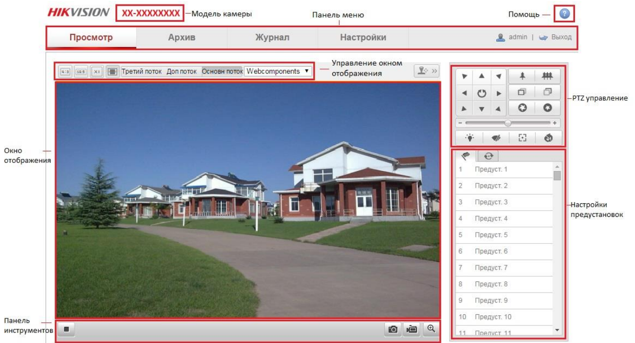
Рисунок 5-1 Интерфейс отображения
