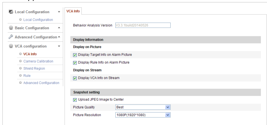
Рисунок 6-48 Анализ поведения
