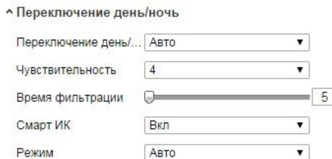
Рисунок 6-24 День/ночь переключение
