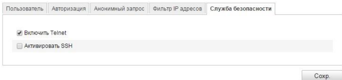
Рисунок 11-8 Служба безопасности
