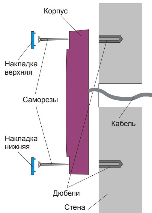
Рисунок 2. Крепление PR-P16
