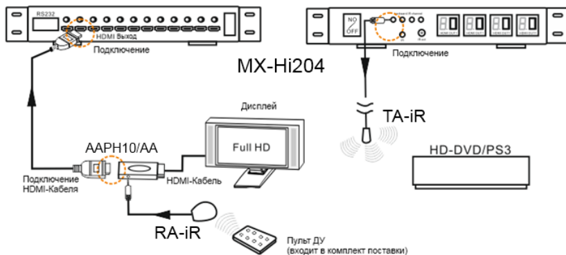
Рис. 4 Схема передачи ИК сигналов коммутатором MX-Hi204
