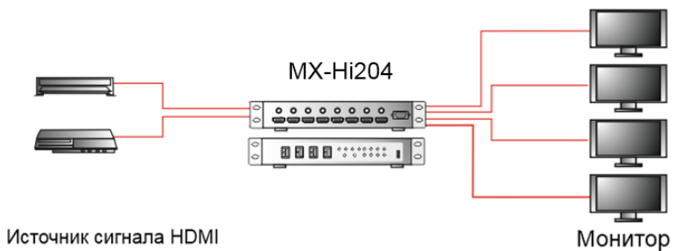
Рис. 3 Схема подключения устройства MX-Hi204
