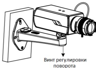
Рисунок 2-8 Установка камеры на кронштейн
