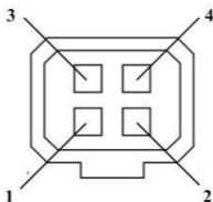
Рисунок 1-4 Auto-iris интерфейс
