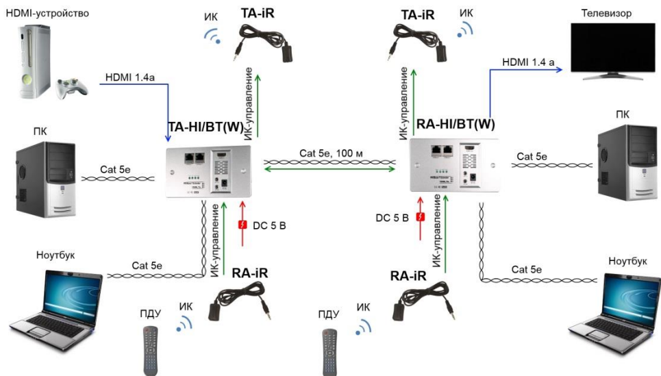
Рис. 3 Схема подключения TA-Hi/VT+RA-Hi/VT / TA-Hi/VT(W)+RA-Hi/VT(W)
