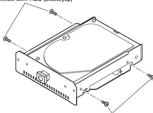
Крепежный винт HDD (аксессуар)
