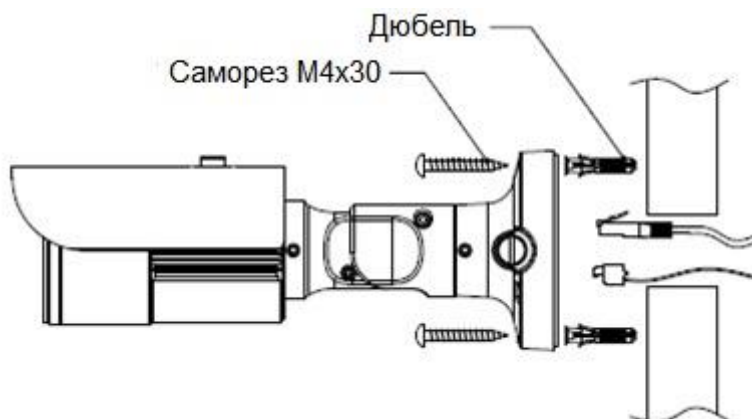
Рис.3.1.1. Монтаж видеокамеры LTV-ICDM*-623LH-V3-9 на потолок / стену
