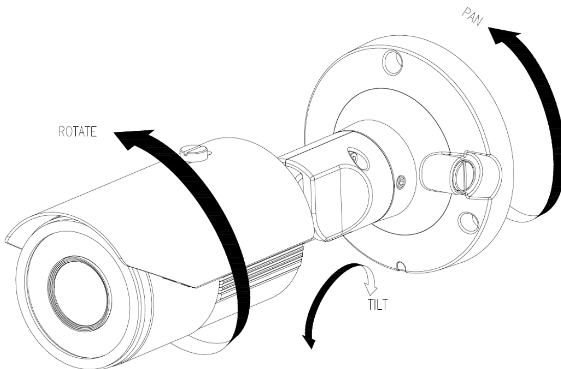
Рис.4.3.1. Предварительная настройка положения видеочамеры LTV-ICDM*-623LH-V3-9
