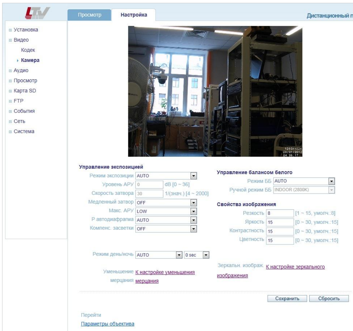
Рис.7.2.1. Меню «Камера»
