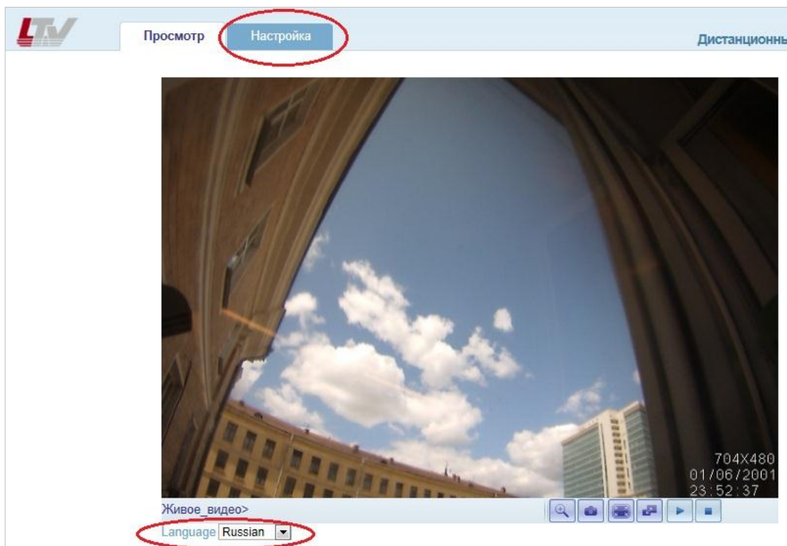
Рис.5.1. Меню «Настройка»
