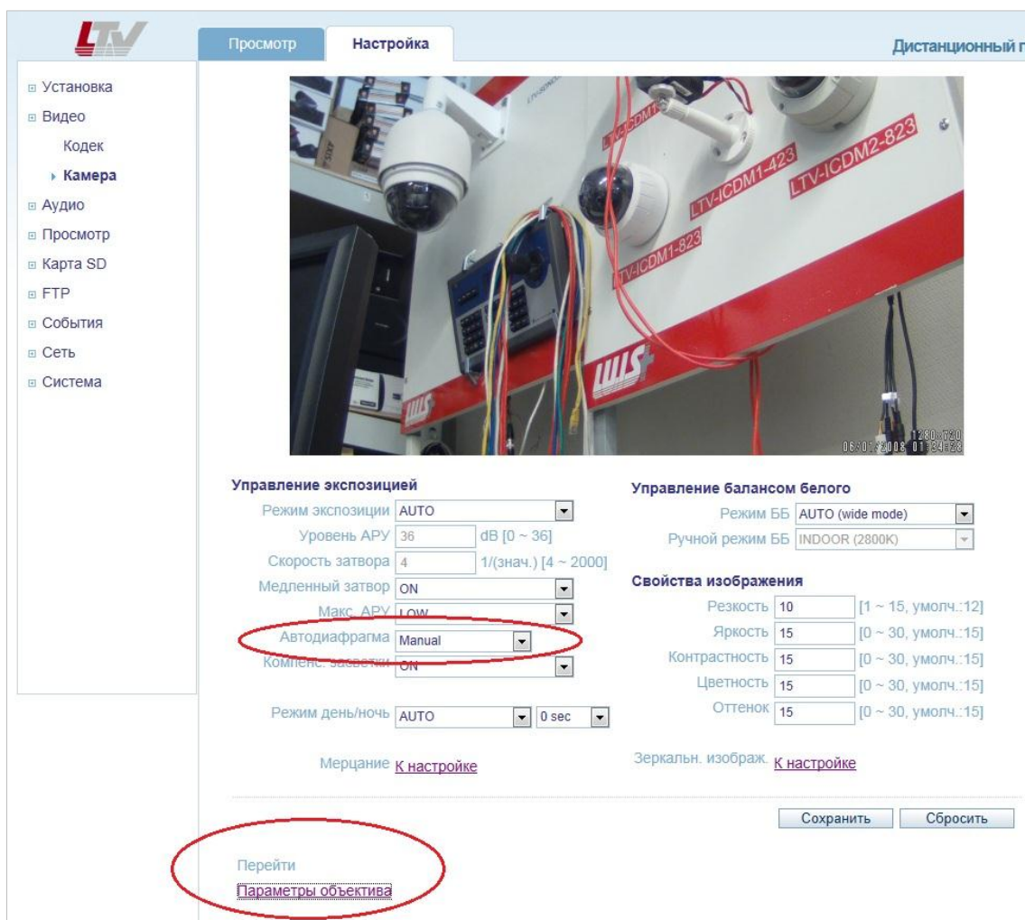
Рис.4.4.1. Меню «Камера»
