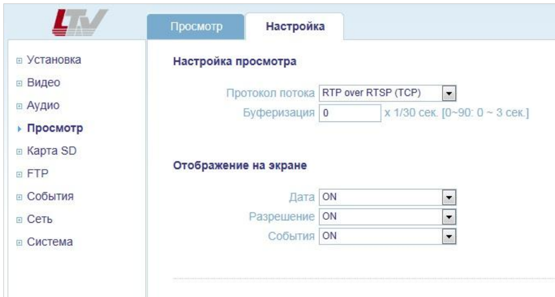
Рис.9.1. Меню «Просмотр»
