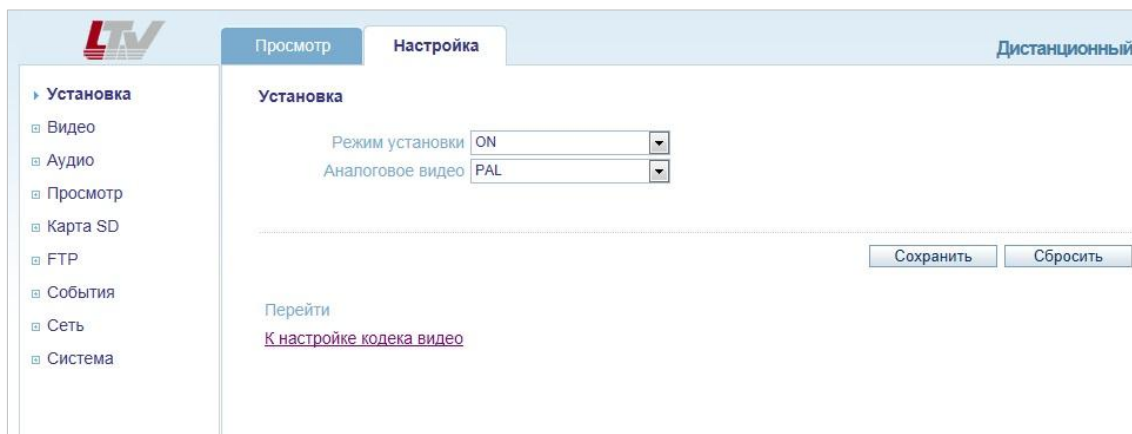
Рис.4.4.3. Меню «Установка»
