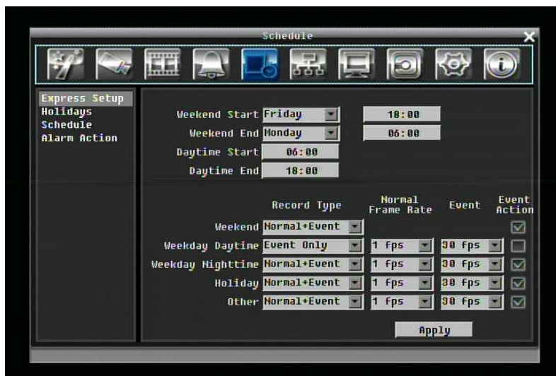
Рисунок 5-20 Меню Расписания-Экспресс Меню
