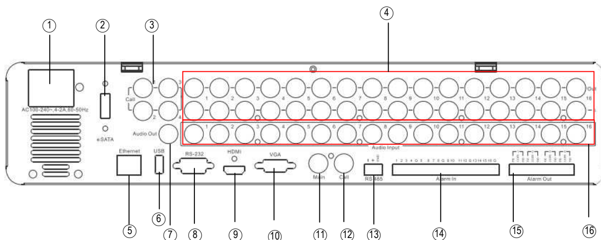
Рисунок 1-2 Задняя Панель
