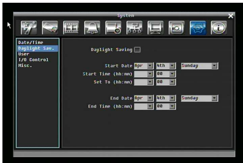
Рисунок 5-35 Меню Системы – Летнее Время
