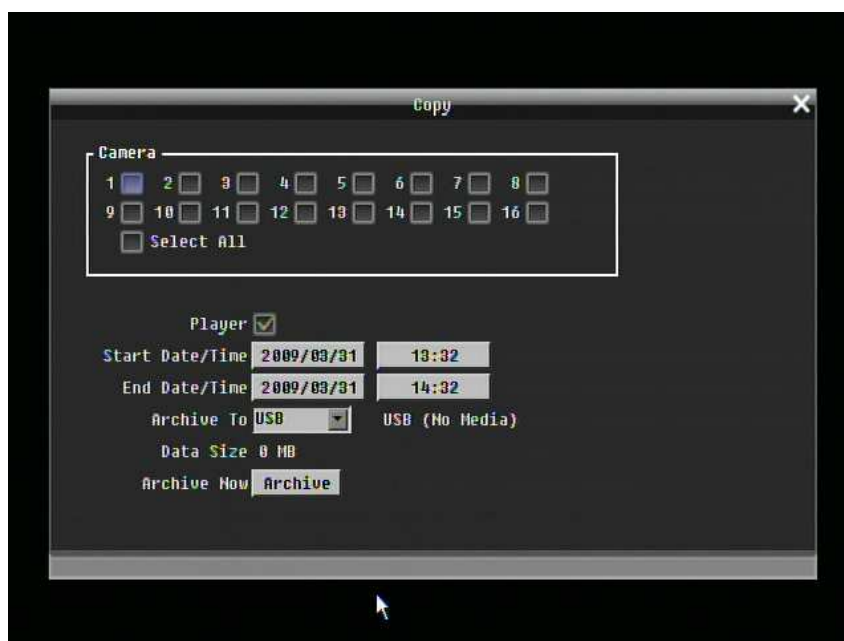
Рисунок 4-9 Меню Копирования
