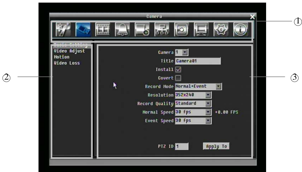
Рисунок 3-3 (Меню OSD)
