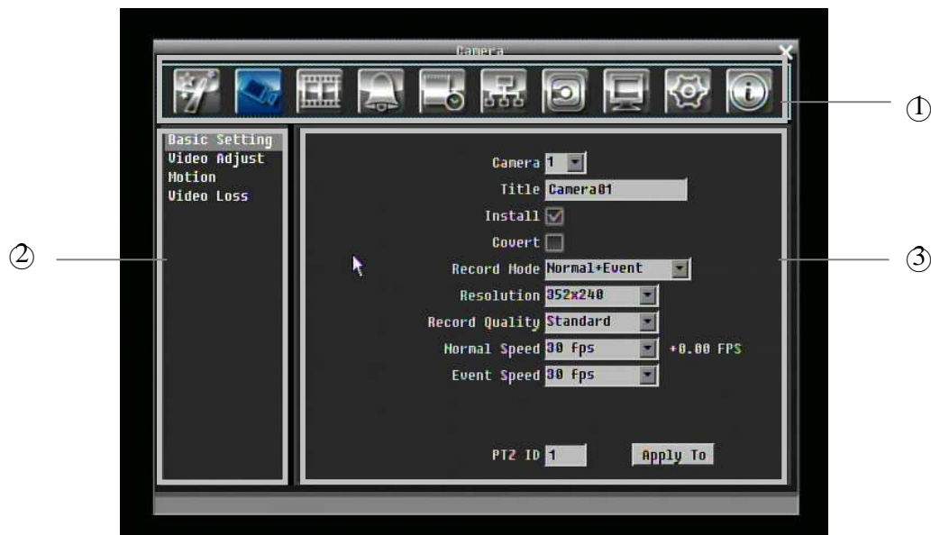
Рисунок 3-2 Меню OSD
