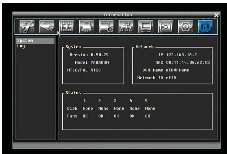
Рисунок 5-41 Меню Информации – Система
