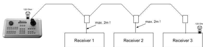
Серия шины RS-485 подключенная с помощью соединительных коробок
