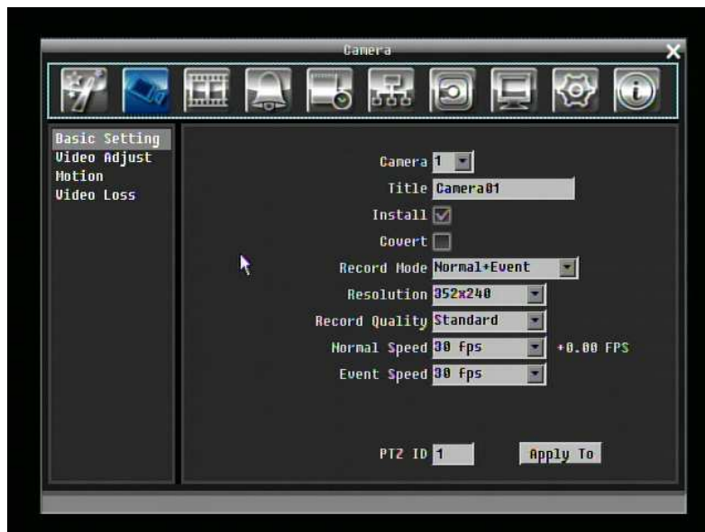
Рисунок 5-2 Меню Камеры-Основные Настройки
