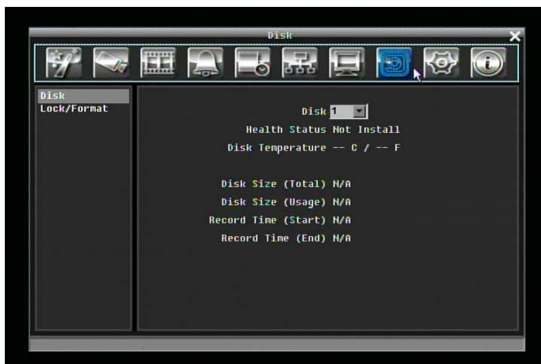
Рисунок 5-32 Меню Диска
