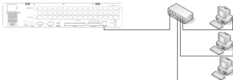
Рисунок 2-2 Сетевое Соединение
