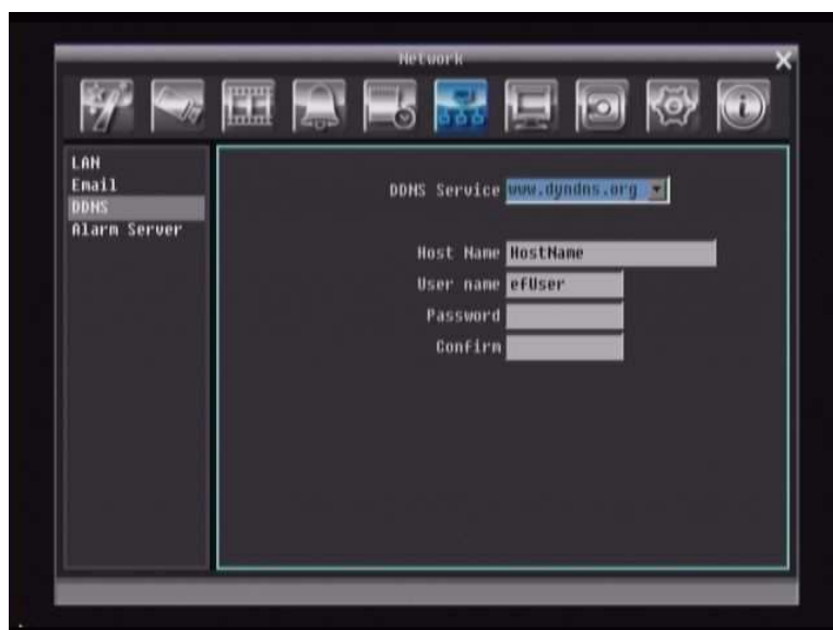
Рисунок 5-27 www.dyndns.org
