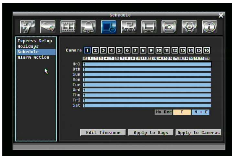
Рисунок 5-22 Меню Расписания-Расписание
