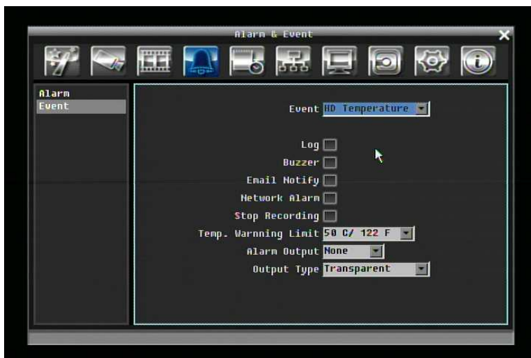
Рисунок 5-13 Меню Тревоги и События – Событие – Температура HD
